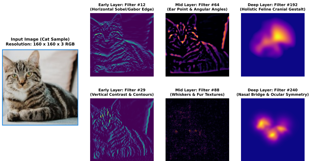
รูปที่ 5: การถอดรหัสฟีเจอร์ภายในโครงข่าย: วิวัฒนาการของ Receptive Field ตั้งแต่เลเยอร์ระดับต้น ( block_1_expand_relu : ตรวจจับเส้นขอบ) ระดับกลาง ( block_13_expand_relu : ตรวจจับลวดลายขนและมุม) จนถึงระดับลึก ( out_relu : ตรวจจับอวัยวะสำคัญบนใบหน้า)
